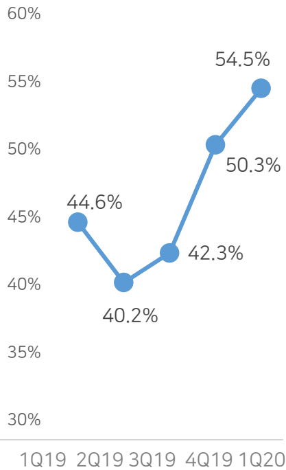
유동 비율 (%)
