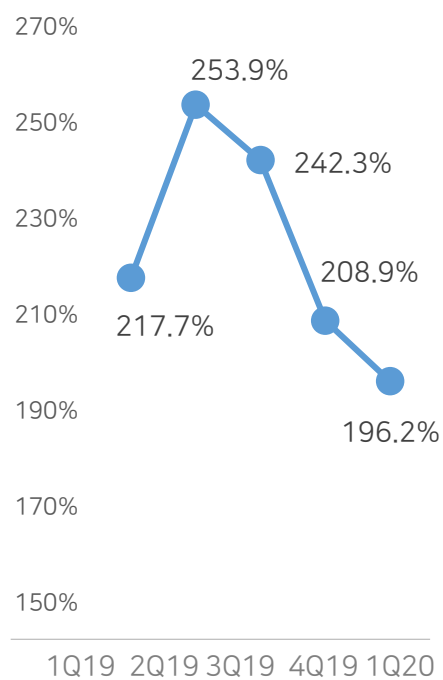
부채 비율 (%)
