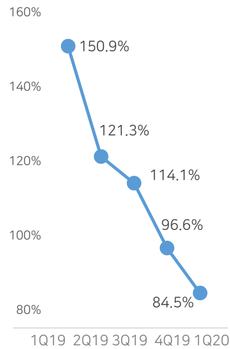
순차입율 (%)
